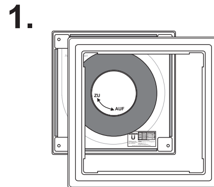
1. Korrekturrahmen unter dem Gehäusedeckel ansetzen.
