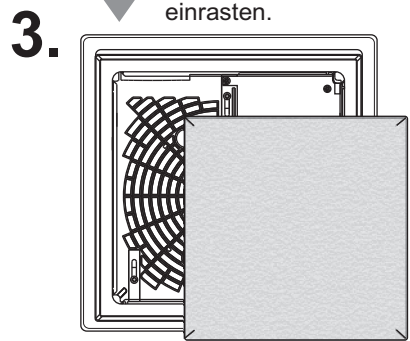
3. Filter in den Gehäusedeckel einlegen (Beschriftungsseite oder farbige Seite nach innen).
